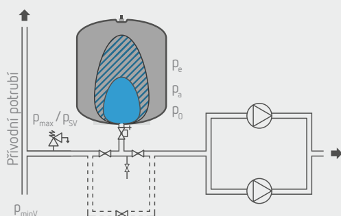
Refix v zařízeních zvyšujících tlak na sací straně
