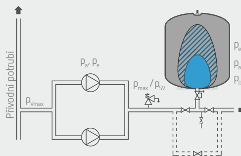
Refix v zařízeních zvyšujících tlak na výtlačné straně
