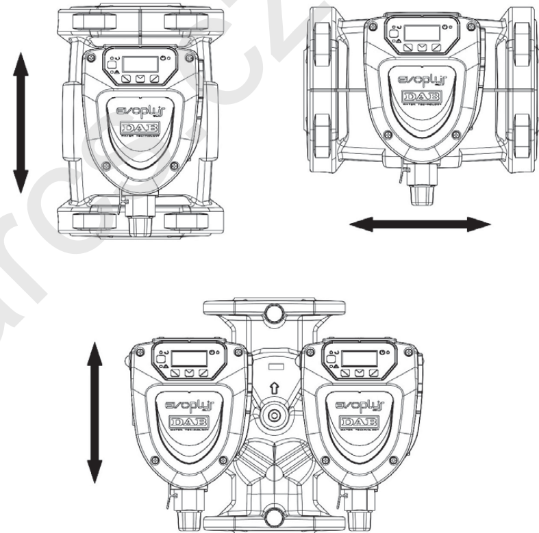
Obr. 1: Montážna poloha
