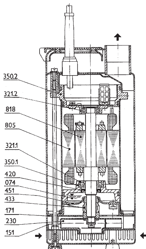
Jednostupňové provedení
